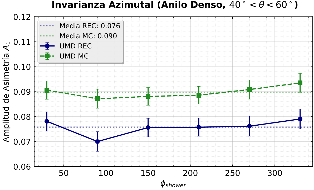
Figura 5.2: Amplitud A_1 en función del ángulo azimutal de la lluvia. Se observa la independencia del observable respecto a la dirección de arribo.
